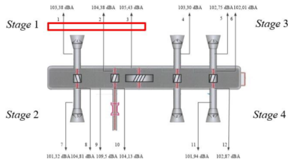
Gambar 2. TTB tiap komponen kompresor (kompresor tampak atas)
