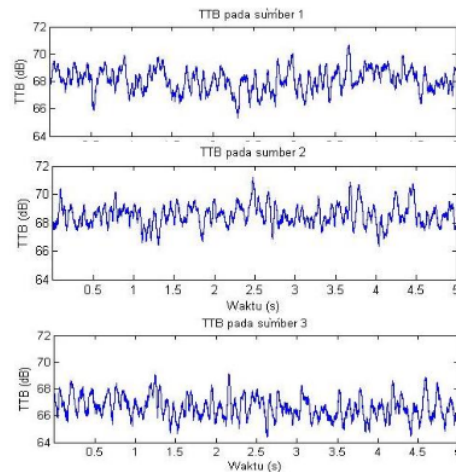
Gambar 6. Tingkat tekanan bunyi tiap sumber bunyi
