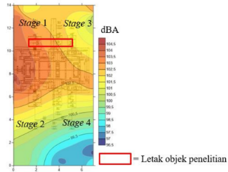
Gambar 1. Noise mapping pada area kompresor
