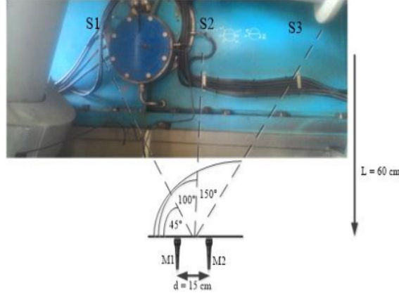
Gambar 3. Pengaturan eksperimen sinyal campuran dengan jarak 60 cm
