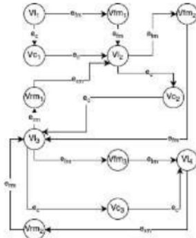
Gambar 4 Model Graf Inter-Struktur dari CD2
