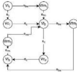
Gambar 3 Model Graf Inter-Struktur dari CD1
