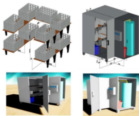
Gambar 3 Rancangan Cold Storage untuk Produk Urban Farming [10]
