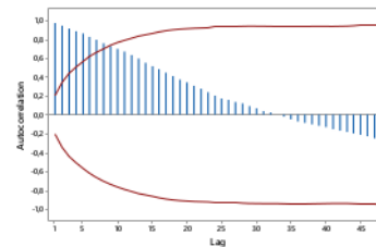
Gambar 6. Plot ACF Provinsi Aceh
