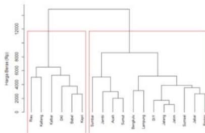
Gambar 9. Diagram Pohon dengan DTW
