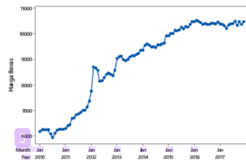
Gambar 5. Plot Harga Beras Provinsi Aceh
