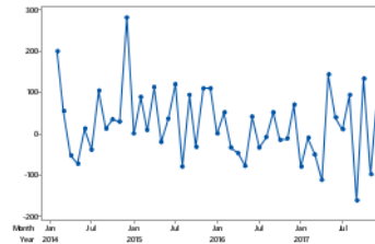
Gambar 7. Plot Pembedaan Pertama Harga Beras di Provinsi Aceh
