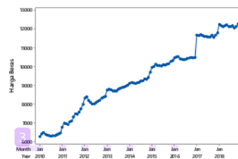
Gambar 2. Pola Harga Beras 6 Provinsi
