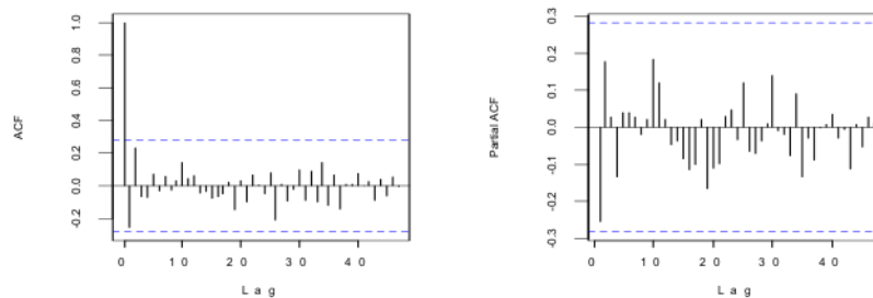
Gambar 8. Plot ACF dan PACF Pembedaan Pertama Harga Beras Provinsi Aceh
